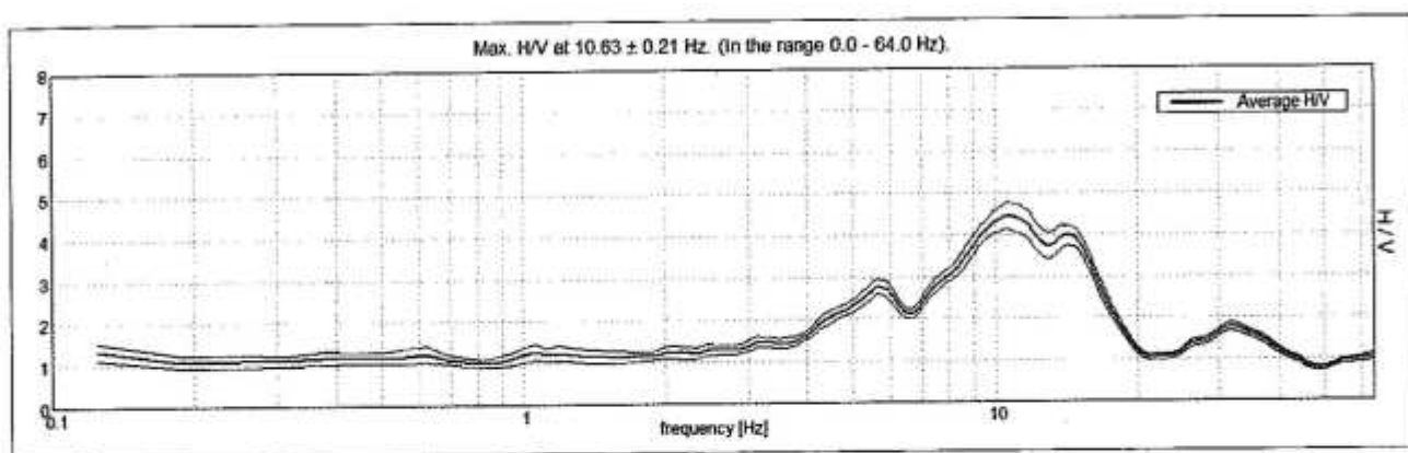
Figura 4: diagramma HVSR relativo alla misura Tr1
