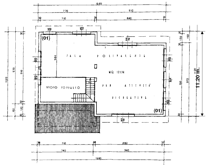
PIANO PRIMO (02)
