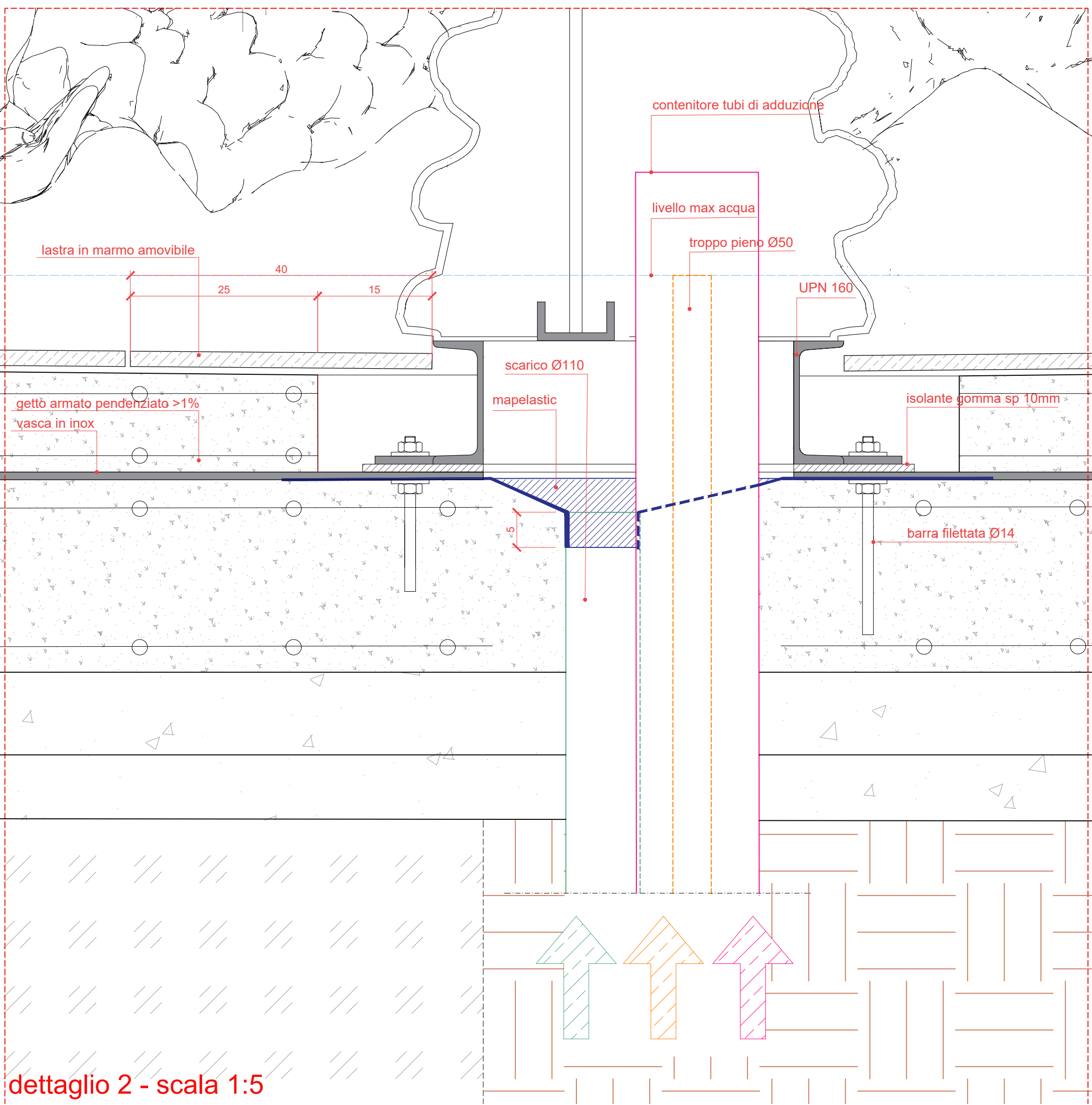
dettaglio 2 - scala 1:5
