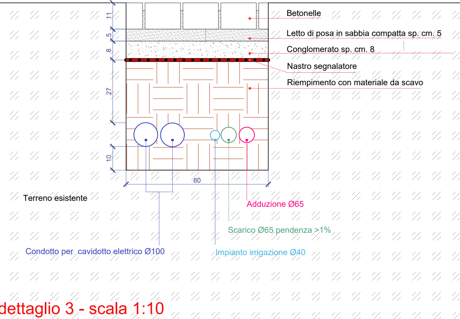
dettaglio 3 - scala 1:10
